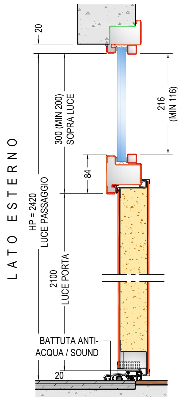
SEZIONE VERTICALE PORTA MODELLI "B-C-D-E" rif. PORTA H=2100 - SOPRA LUCE 300 LUCE PASSAGGIO HP=2420
