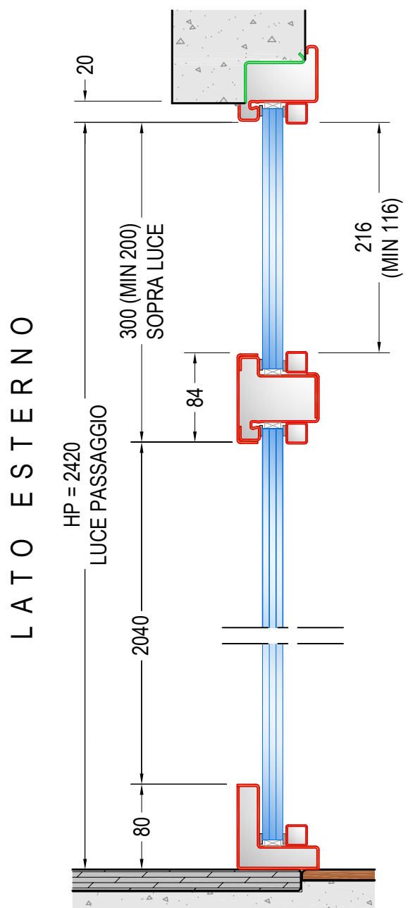
SEZIONE VERTICALE FIANCO LUCE MODELLI "C-D-E" rif. PORTA H=2100 - SOPRA LUCE 300 LUCE PASSAGGIO HP=2420
