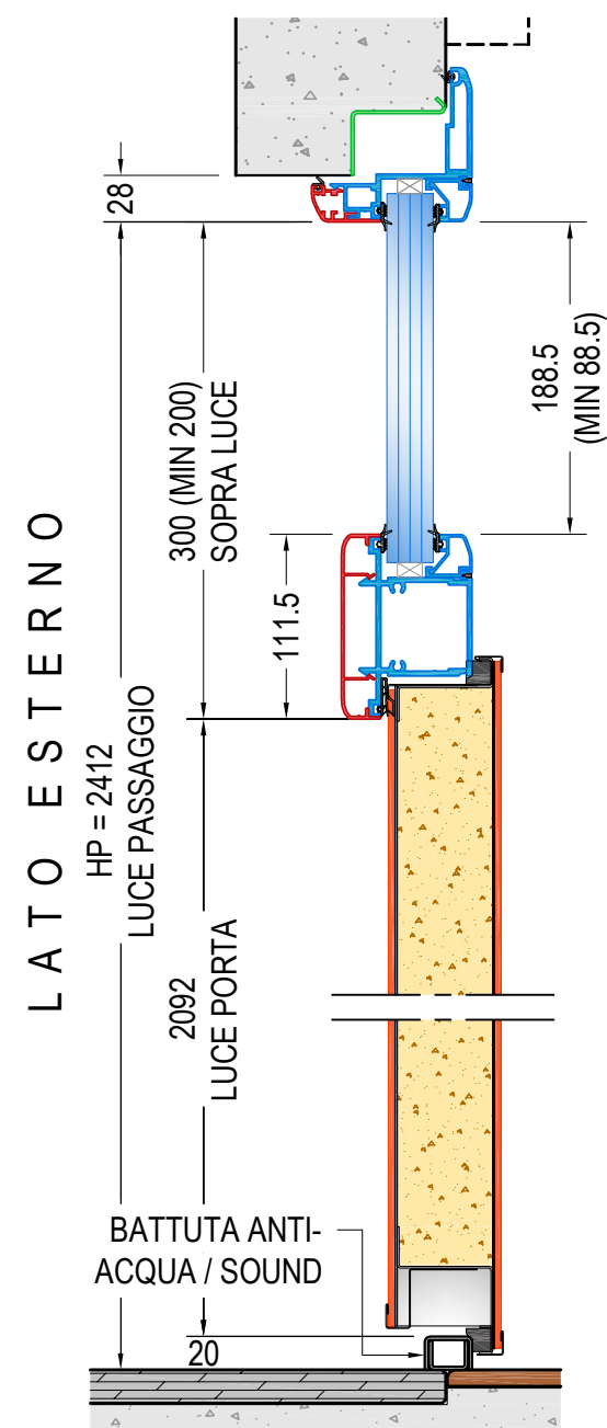
SEZIONE VERTICALE PORTA MODELLI "B-C-D-E" rif. PORTA H=2100 - SOPRA LUCE 300 LUCE PASSAGGIO HP=2412
