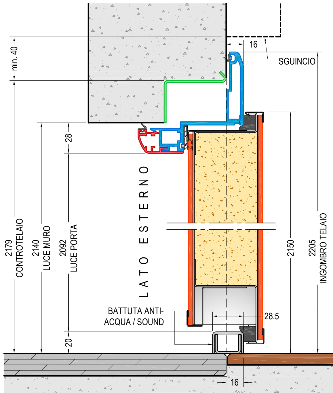
SEZIONE VERTICALE PORTA MODELLI "A-F-G-H" rif. PORTA H=2100
