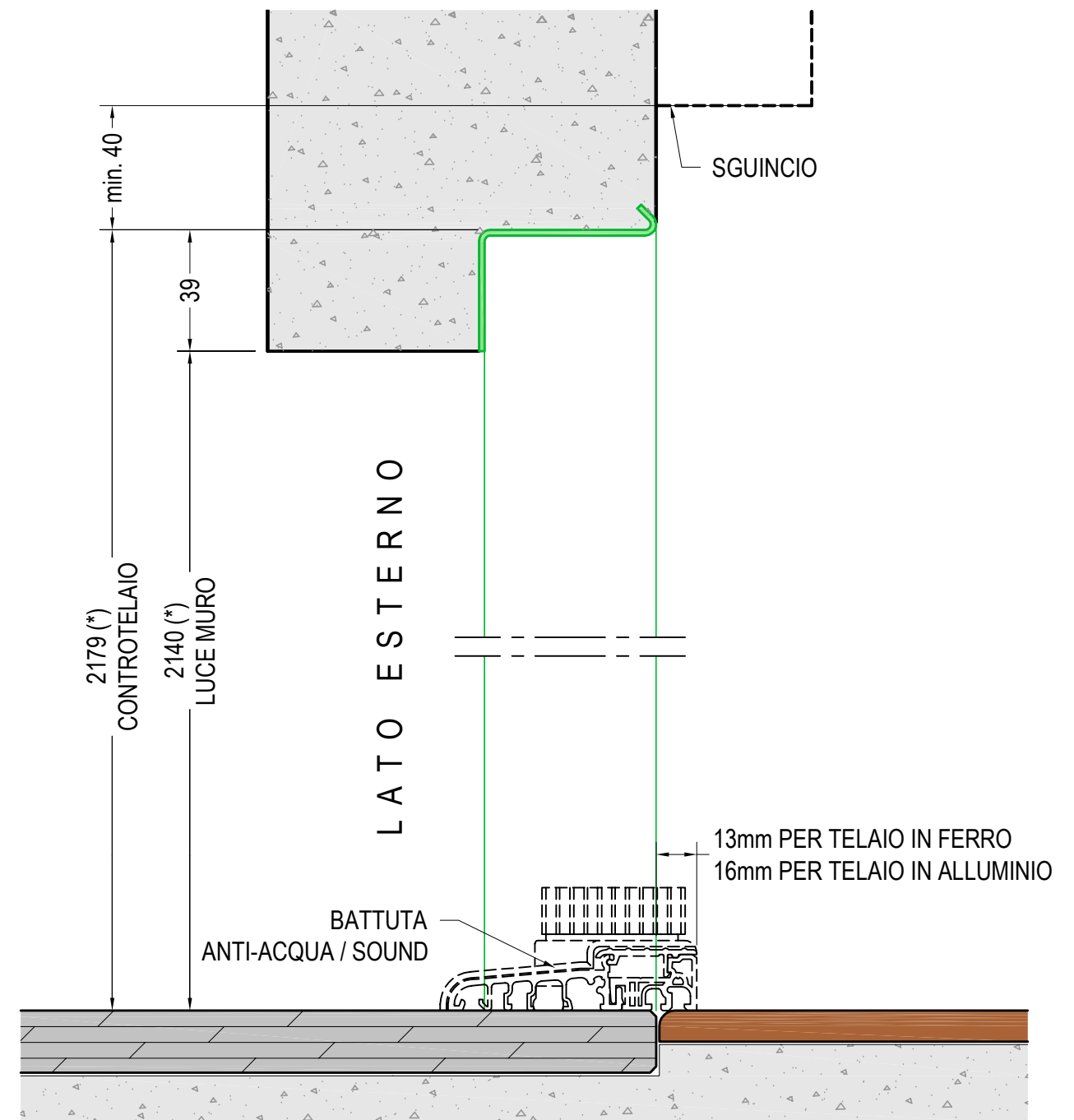
SEZIONE VERTICALE rif. PORTA H=2100
