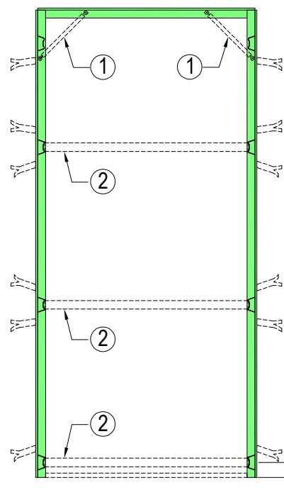
VISTA LATO INTERNO
