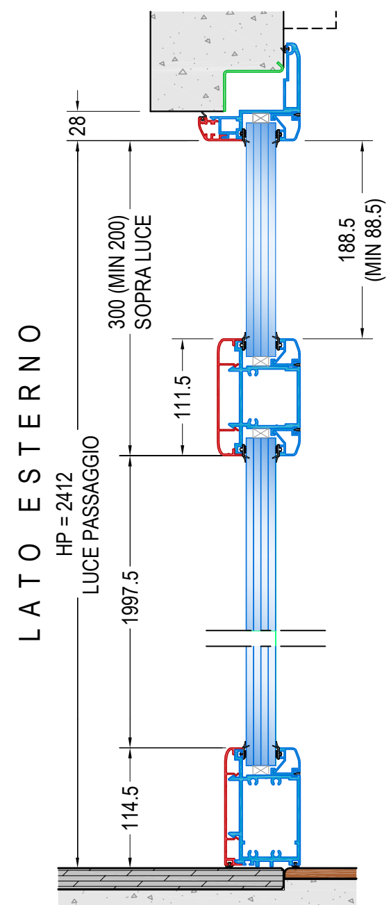
SEZIONE VERTICALE FIANCO LUCE MODELLI "C-D-E" rif. PORTA H=2100 - SOPRA LUCE 300 LUCE PASSAGGIO HP=2412
